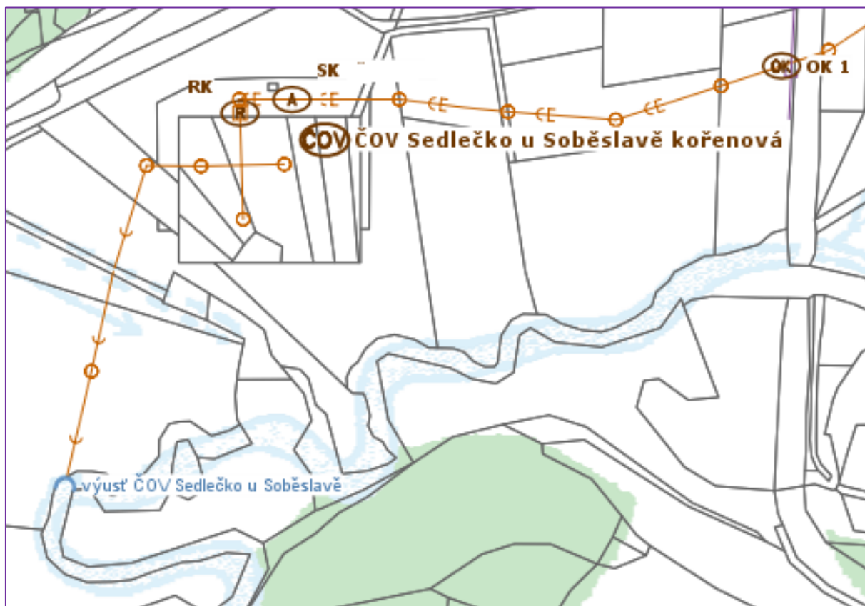
Situace ČOV Sedlečko u Soběslavě :
